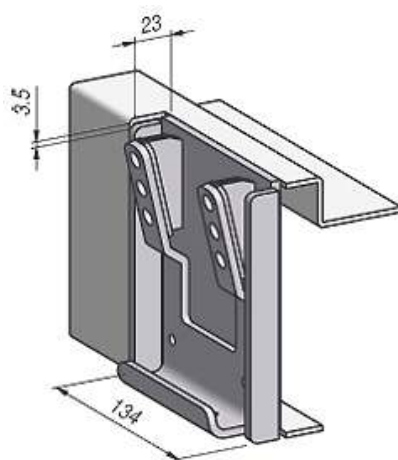
Soporte Kinnegrip K-20 para soldar 026 020 4695
