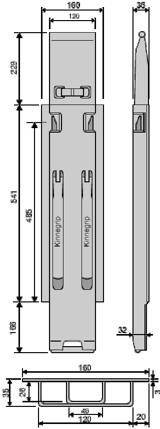
Pilar Kinnetop K-4 en aluminio de 500 (Consultar referencia)
