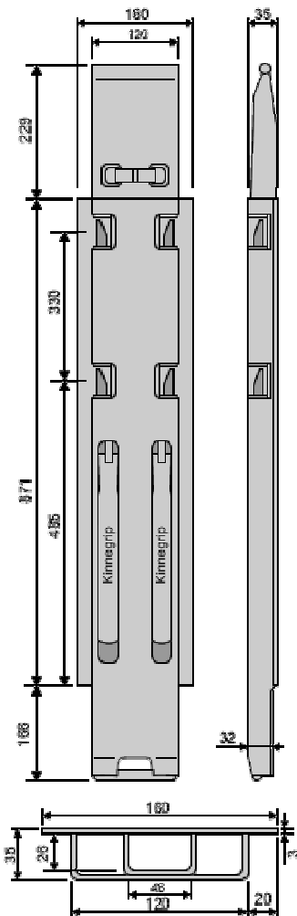
Pilar Kinnetop K-4 en aluminio de 800 026 020 4376
