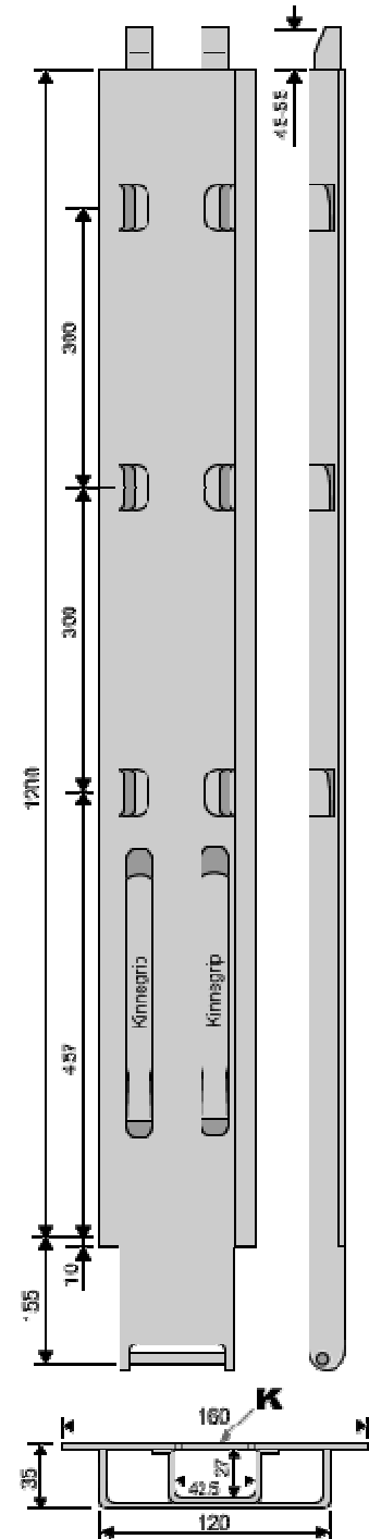
Pilar Kinnetop K-20 de 1200
