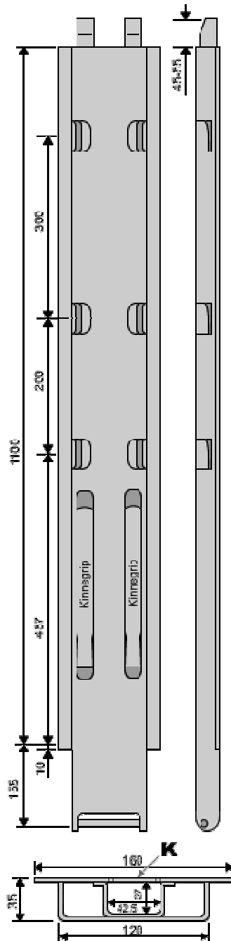
Pilar Kinnetop K-20 de 1100
