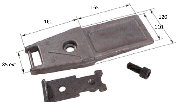
Conjunto de cuña de forja con soporte y tornillo frontal 021 050 2885
