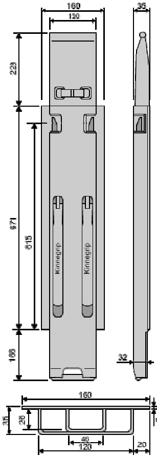
Pilar Kinnetop K-4 en aluminio de 600 026 020 4375
