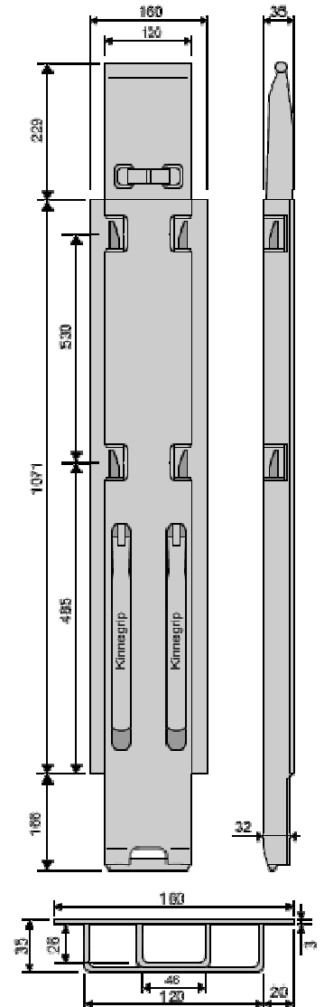
Pilar Kinnetop K-4 en aluminio de 1000 026 020 4376
