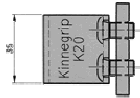
Gancho completo Kinnetop K-20 026 020 3065
