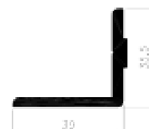
L para lateral (18585) 005 020 0705 (L=6,2 m)
