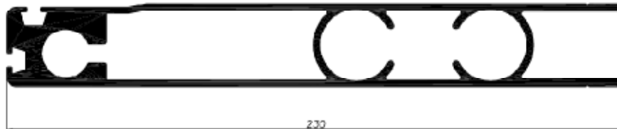
Perfil puerta telescópica (16266) 005 020 00974 (L=5,8 m) 005 020 0805 (L=6 m)
