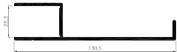
Perfil interior derecho puerta telescópica (17293) 005 020 01722 (L=6 m)
