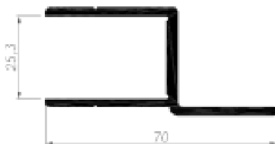
U Ala larga (13235) 005 020 0622 (L=6,2 m)
