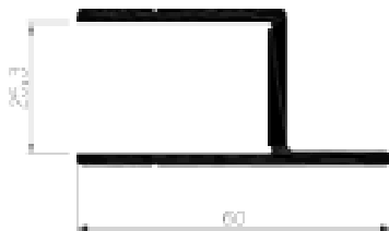
U Ala plana (12925) 005 020 0676 (L=5,1 m)
