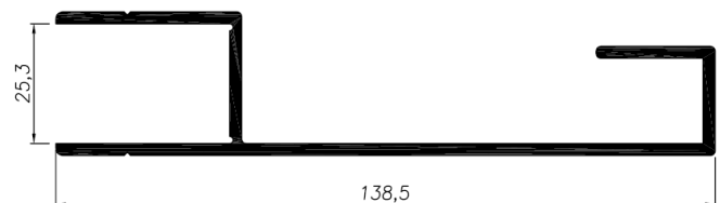
Perfil interior izquierdo puerta telescópica (17292) 005 020 01721 (L=6 m)
