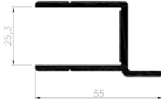
U Ala larga abultada (12926) 005 020 0673 (L=5,1 m)
