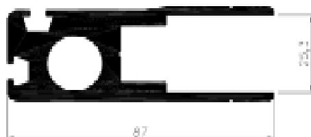
Marco puerta exterior (16269)
