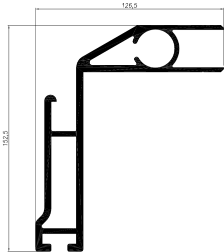
Cantoneira frente (16217) 005 020 0807 (L=6 m) 005 020 01902 (L=5 m)
