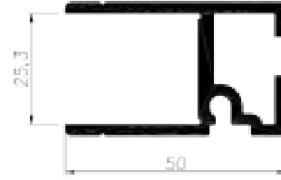
Borde Kinnegrip (12929) 005 020 0657 (L=5,1 m)
