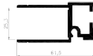
Borde para Kinnegrip K20 (16722) 005 020 0662 (L=5,7 m)
