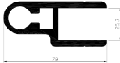
Pilar puerta exterior (16268)
