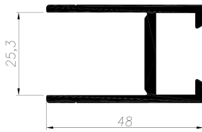
Marco puerta estándar (13082)
