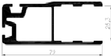
Marco puerta exterior-central (20445)
