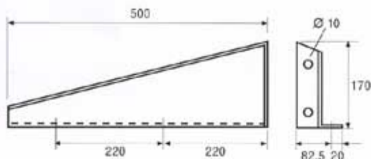
Ref. 2690.32 • Conjunto soporte para depósitos / Peso 1,490 kg. Bracket set for tanks / Weight 1.490 kg.
