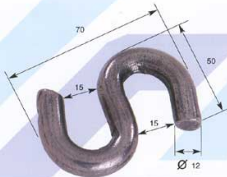
Ref. 2763 • Gancho S de 12 / Peso 0,125 kg. 12 S-hook / Weight 0.125 kg.
